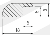
штапик под стекло
