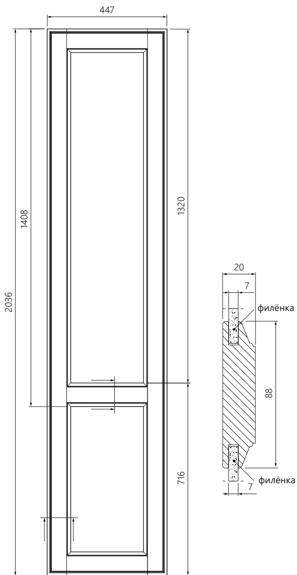
фасад с филёнкой 2036x447 LL
