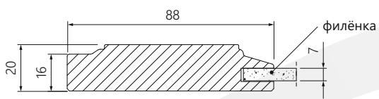
фасад с филёнкой 2036x447 LL
