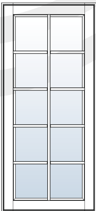
фасад с обрешеткой тип К со стеклом 1316x597 VLG
