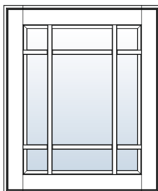
фасад с обрешеткой тип А со стеклом 956x597 VLG
