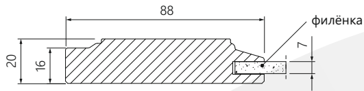
фасад с филёнкой
