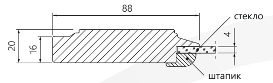
фасад со стеклом
