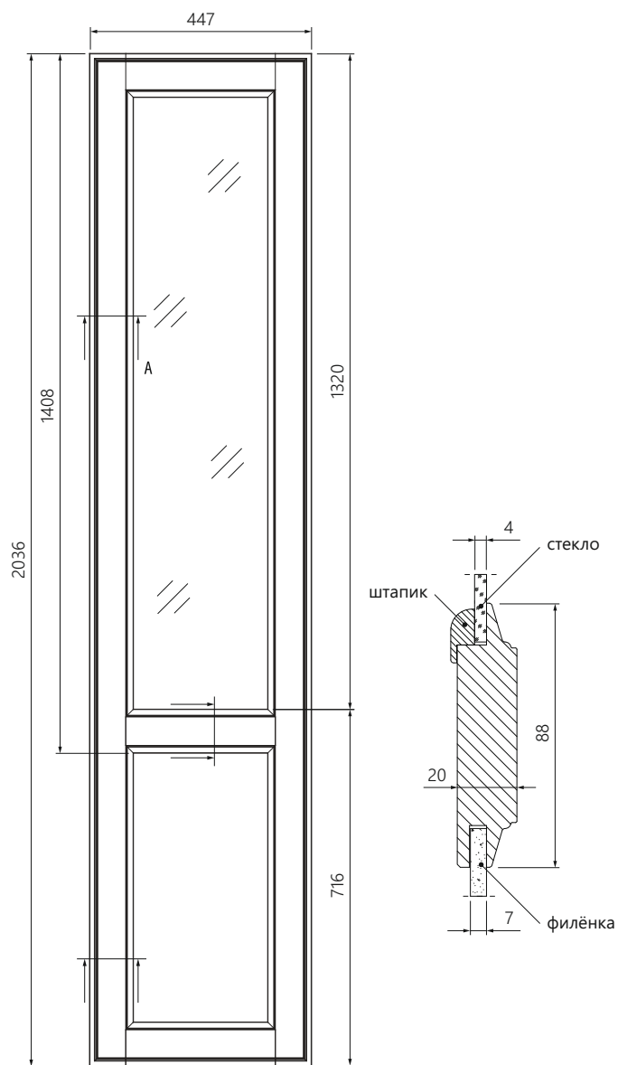
фасад со стеклом/филёнкой 2036x447 VL
