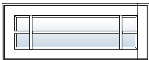
фасад с обрешеткой тип А со стеклом 896x597 VLG
