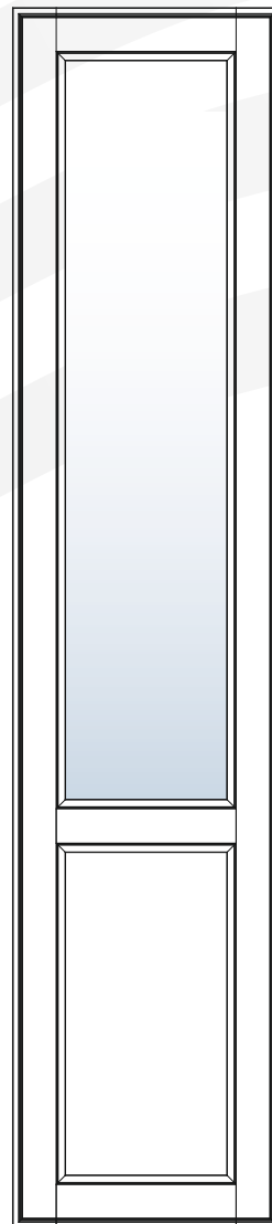
фасад со стеклом/филенкой 2036x447 UL
