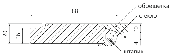
фасад с обрешеткой тип А со стеклом
