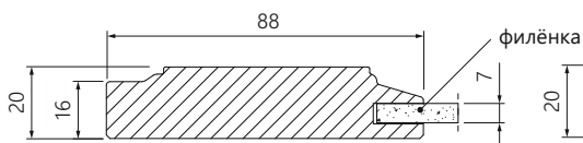
накладка на ящик 177x447
