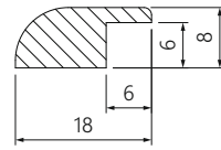
штапик под стекло и решетку
