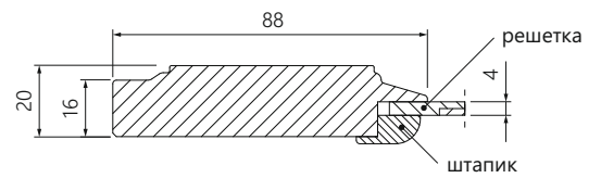
фасад с решеткой №1
