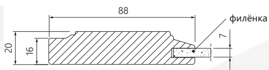
фасад со стеклом/филёнкой 2036x447 VL
